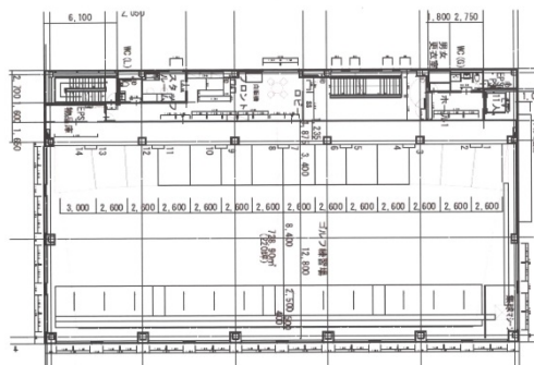
3階区画平面図
