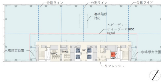
平面図(3・4階) 事務所 1,612㎡ (487.63坪)
