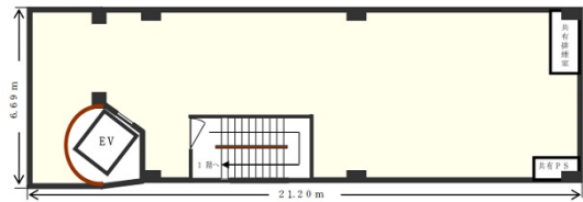
「地下1階平面図」
