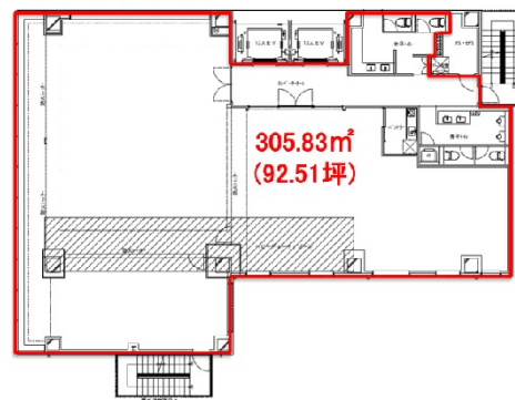
11F 平面図
