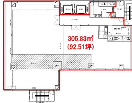
9-10F 平面図
