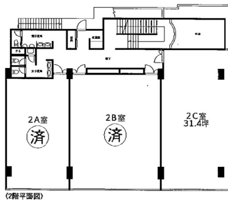
(2階平面図)
