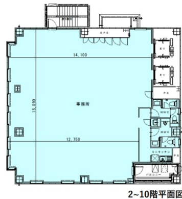
2~10階平面図
