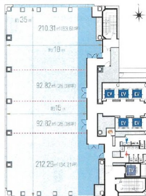
高層基準階平面図 (13F~15F) 608.25㎡ 183.96坪
