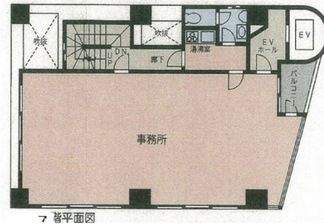
7階平面図
