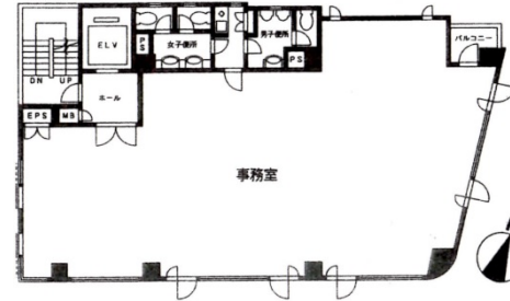
2階平面図
