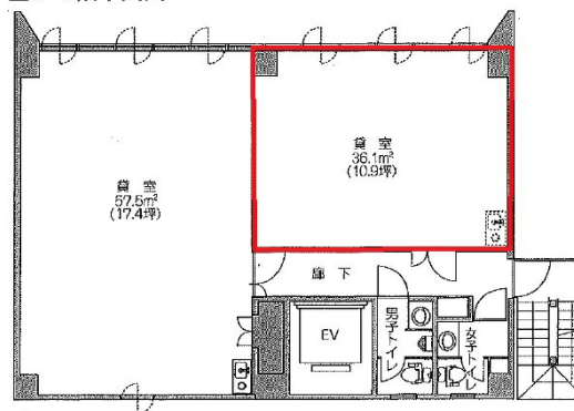
■3~5階平面図
