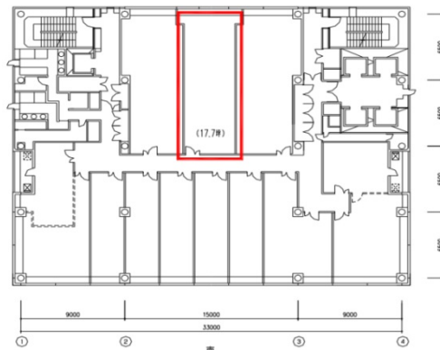
13階 平面図
