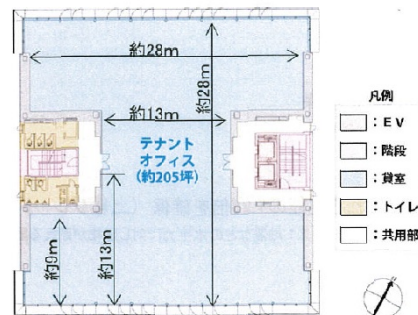
基準階(3-7階)
