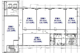
5F 平面図
