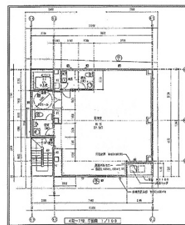
〈4/5/6/7階平面図〉
