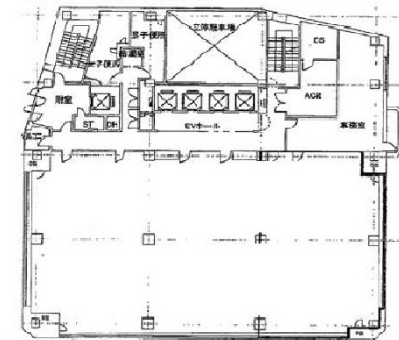
■4～10階平面図
