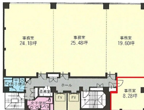
2～6階平面図
