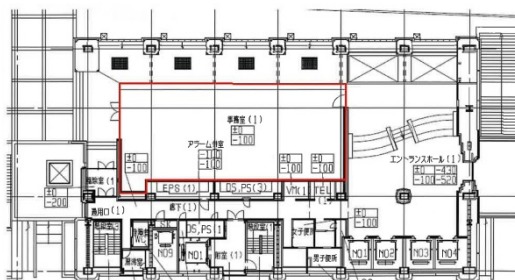
【2階 平面図】
