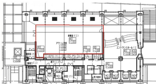
【2階 平面図】
