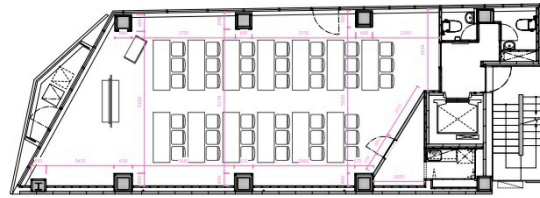
5F平面図
