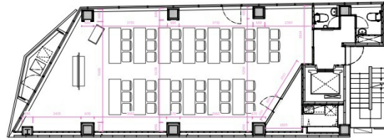
5F平面図
