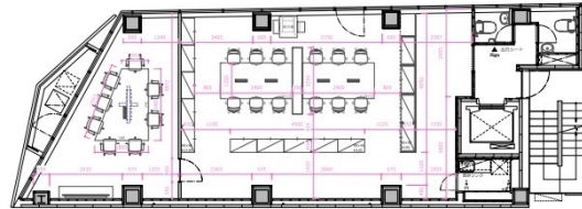
4F平面図
