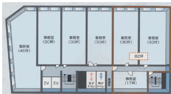
基準階 (2F~5F)
