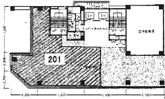
2F 平面図
