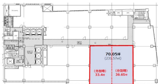
3階 平面図
