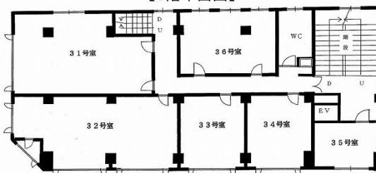
【3階平面図】
