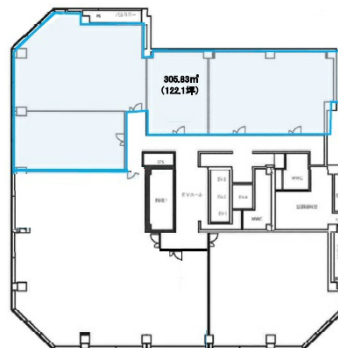
4階平面図
