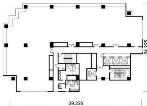
基準階
