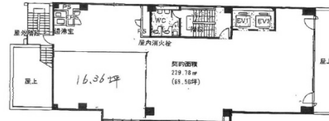
6階平面図
