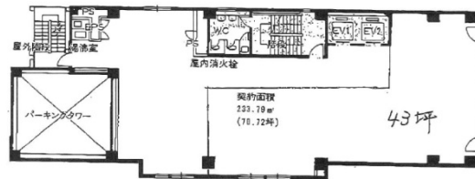
2階平面図
