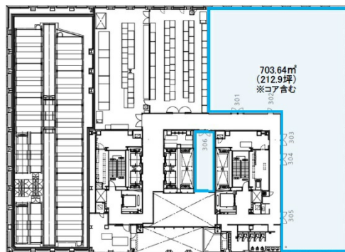
3階平面図
