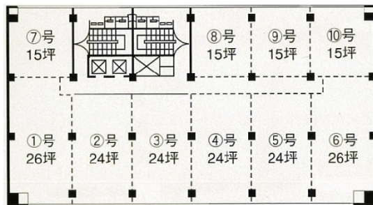
【2階～9階平面図】
