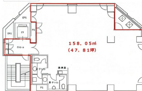
6階平面図
