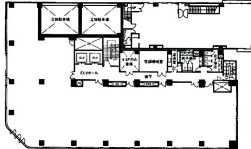
基準階2～6F
