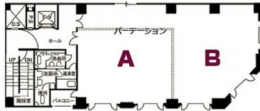
2~8階平面図
