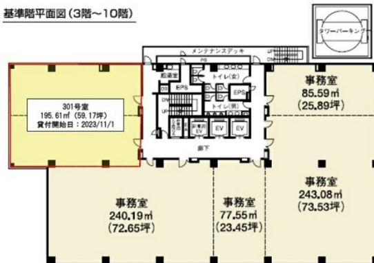
基準階平面図(3階~10階)
