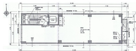
2〜5階平面図
