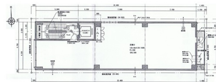
2～5階平面図
