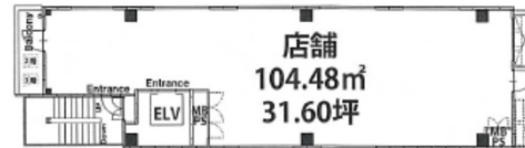
2～9階平面図
