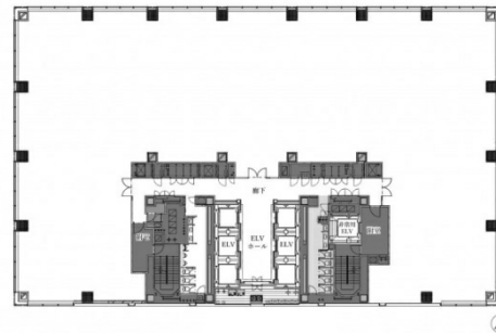
基準階357.36坪
