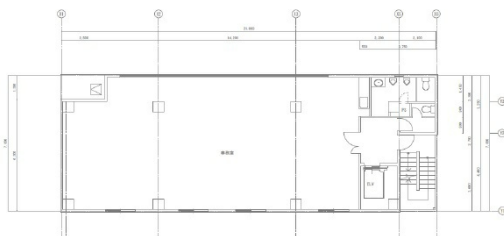
【2～5階平面図】
