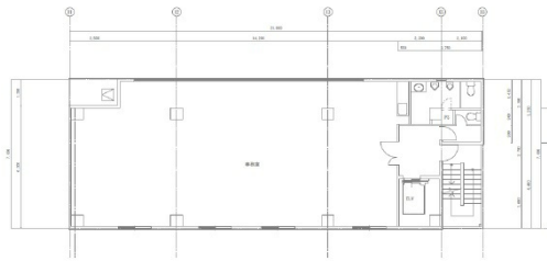
【2～5階平面図】
