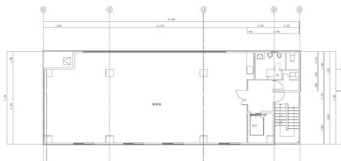
【2～5階平面図】
