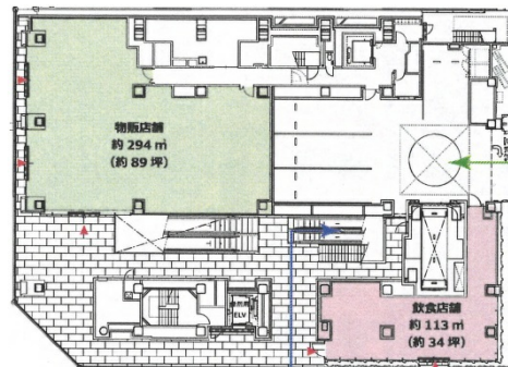
1階平面図
