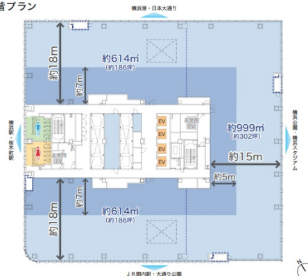
基準階プラン
