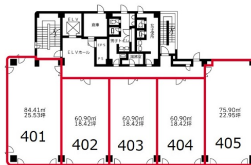
4階平面図
