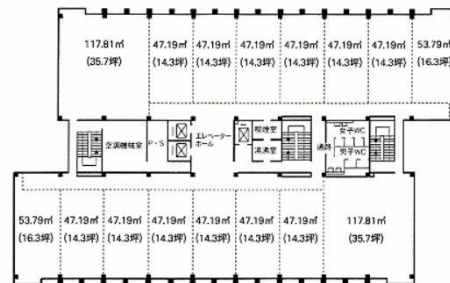
ビル基準平面図
