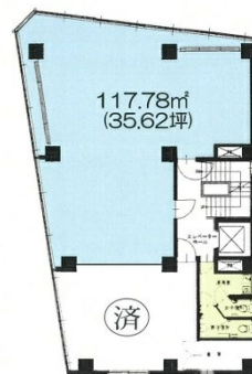
3階平面図
