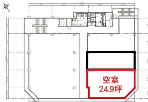
5階平面図
