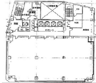
■4～10階平面図
